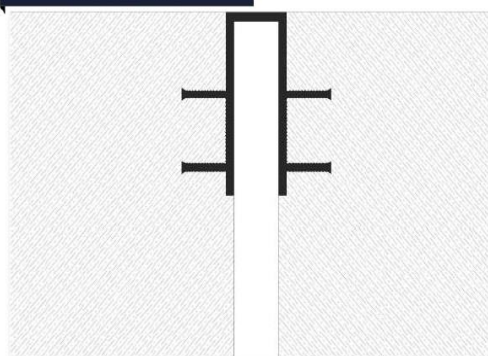
Монтажная схема
